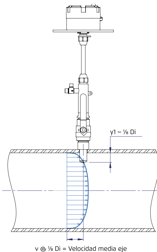
Fig. 57 Principio de funcionamiento
