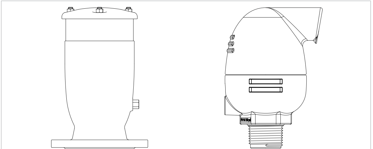
Fig. 42 Válvula combinada típica de alivio de aire, diseñada con funciones de liberación de aire automático y cinético
