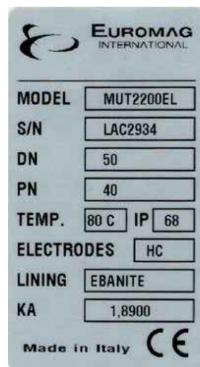
Fig. 1 Placa identificativa
